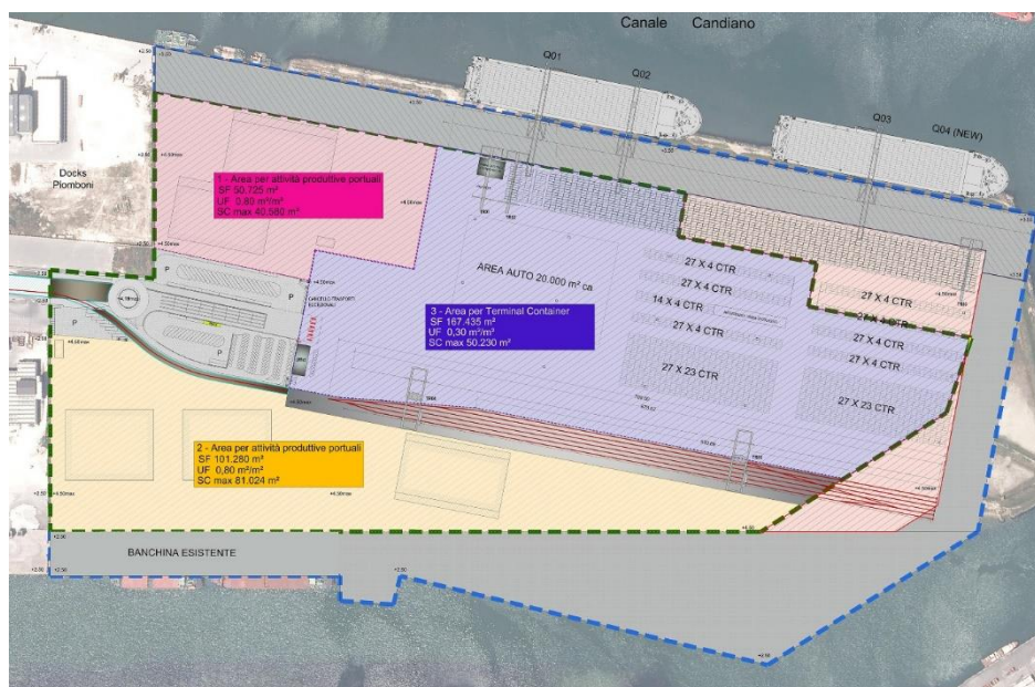
Figura 26 – Nuovo terminal Container. Estratto da Progetto Unitario “Trattaroli Destra”. Fonte: Sapir – Porto Intermodale Ravenna spa
