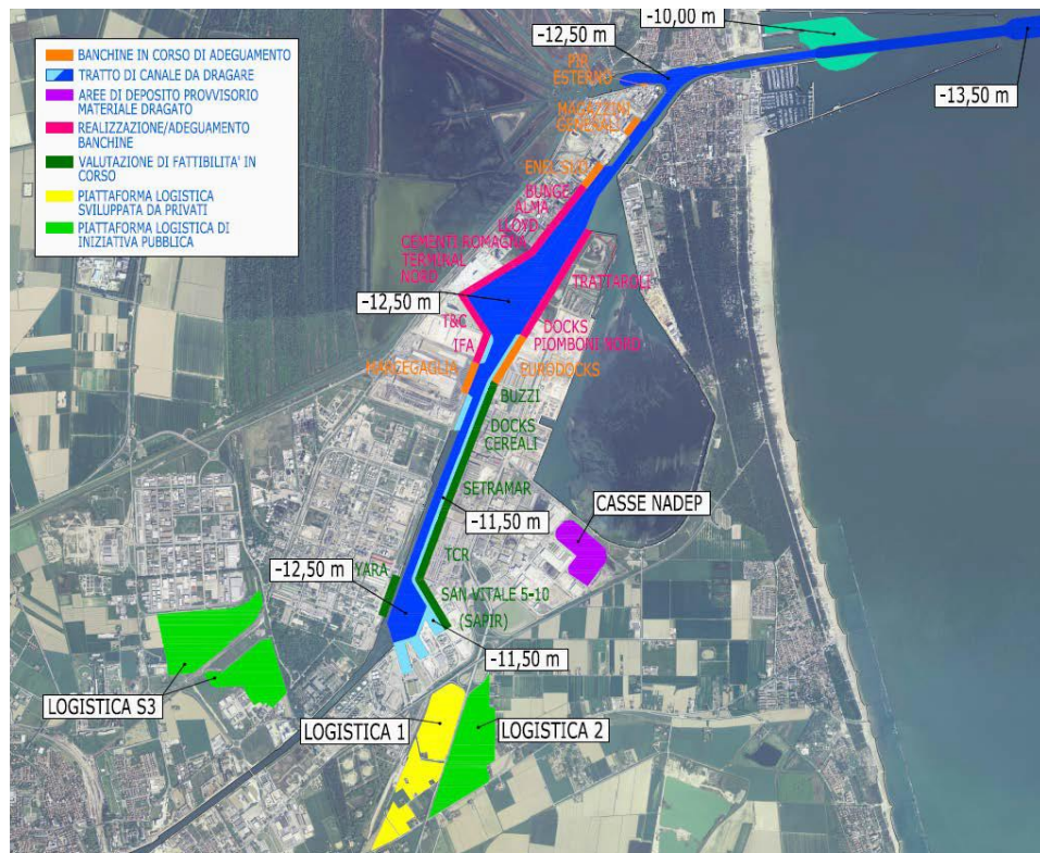
Figura 34 – Inquadratura generale del progetto Hub Portuale di Ravenna - Fonte: AdSP
