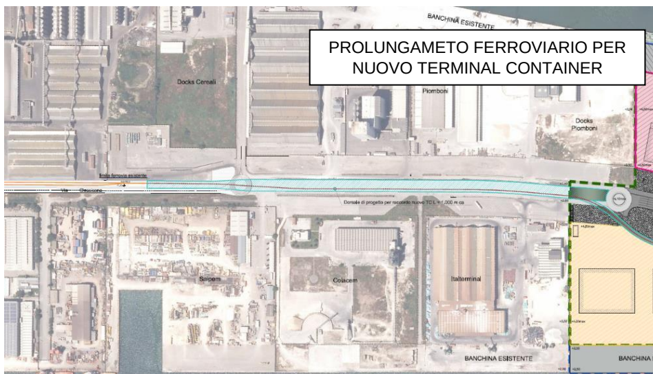
Figura 25 – Raccordo tra attuale termine dei binari e prolungamento verso nuovo terminal Container (in azzurro). Estratto da Progetto Unitario "Trattaroli Destra". Fonte: Sapir – Porto Intermodale Ravenna spa
