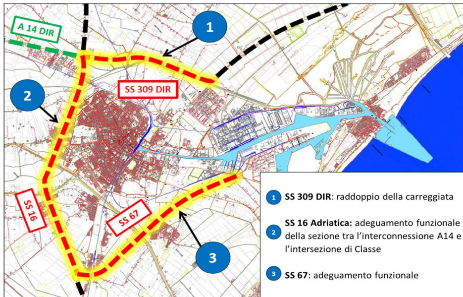
Figura 36 – Interventi previsti per il potenziamento dell'accessibilità stradale - Fonte: AdSP
